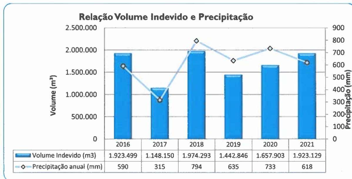
Gráfico 12 – Relação entre o volume indevido e a precipitação
