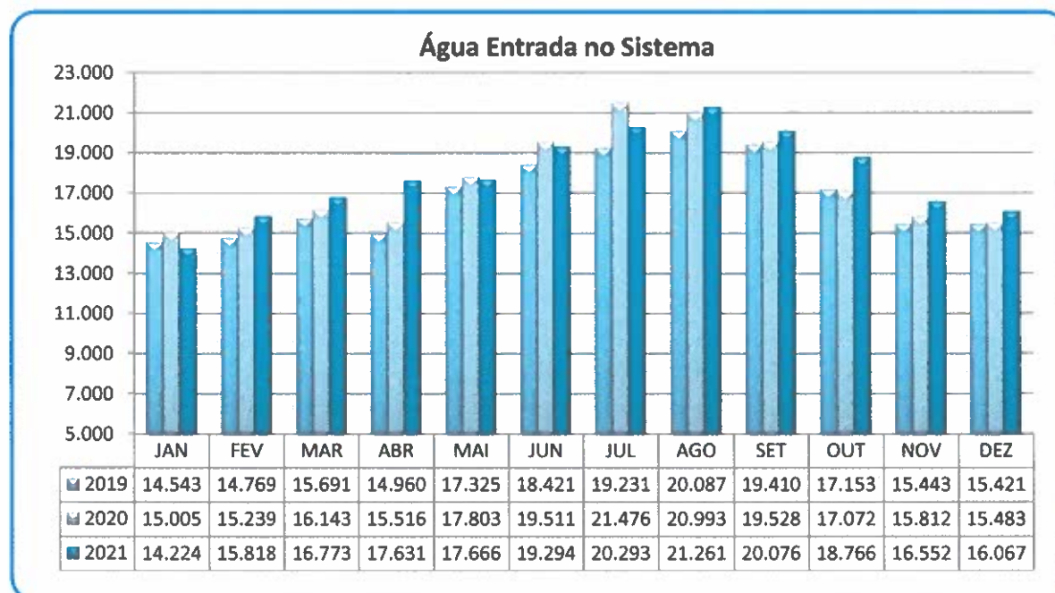
Gráfico 5 – Volume médio diário de água entrada no sistema
