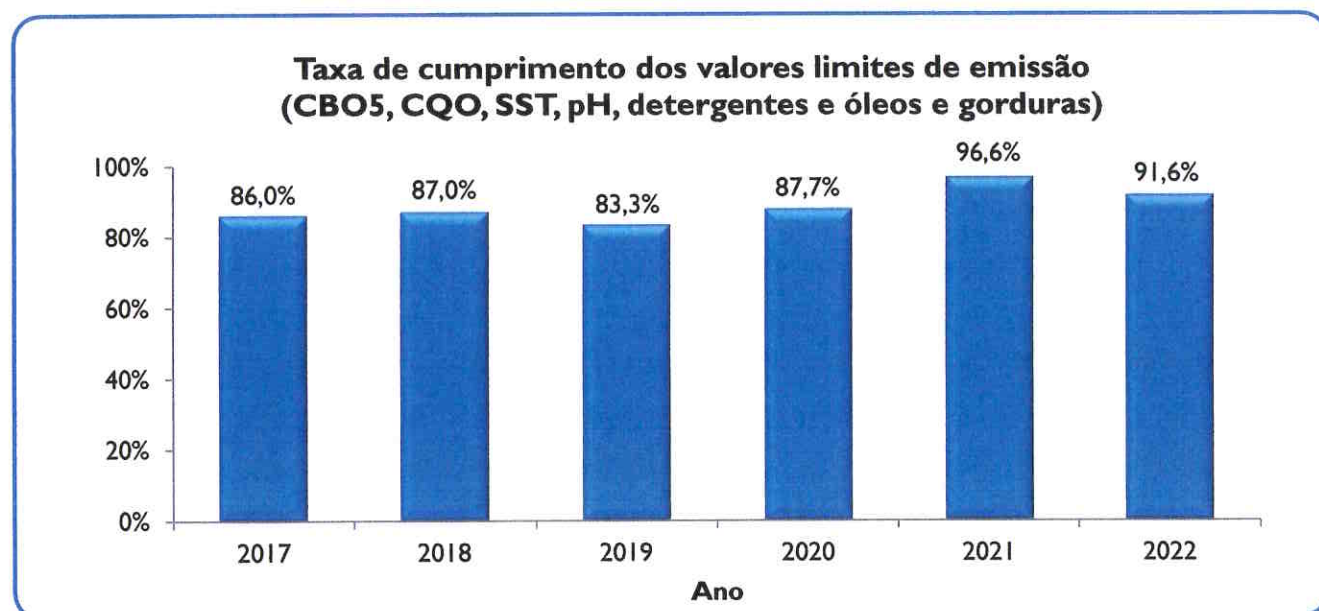
Gráfico 16 - Histórico do cumprimento da taxa dos valores limites de emissão
