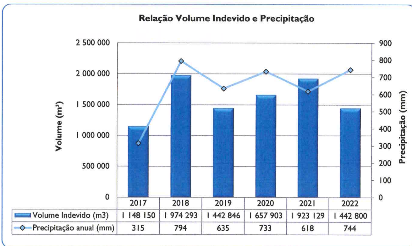
Gráfico 13 – Relação entre o volume indevido e a precipitação
