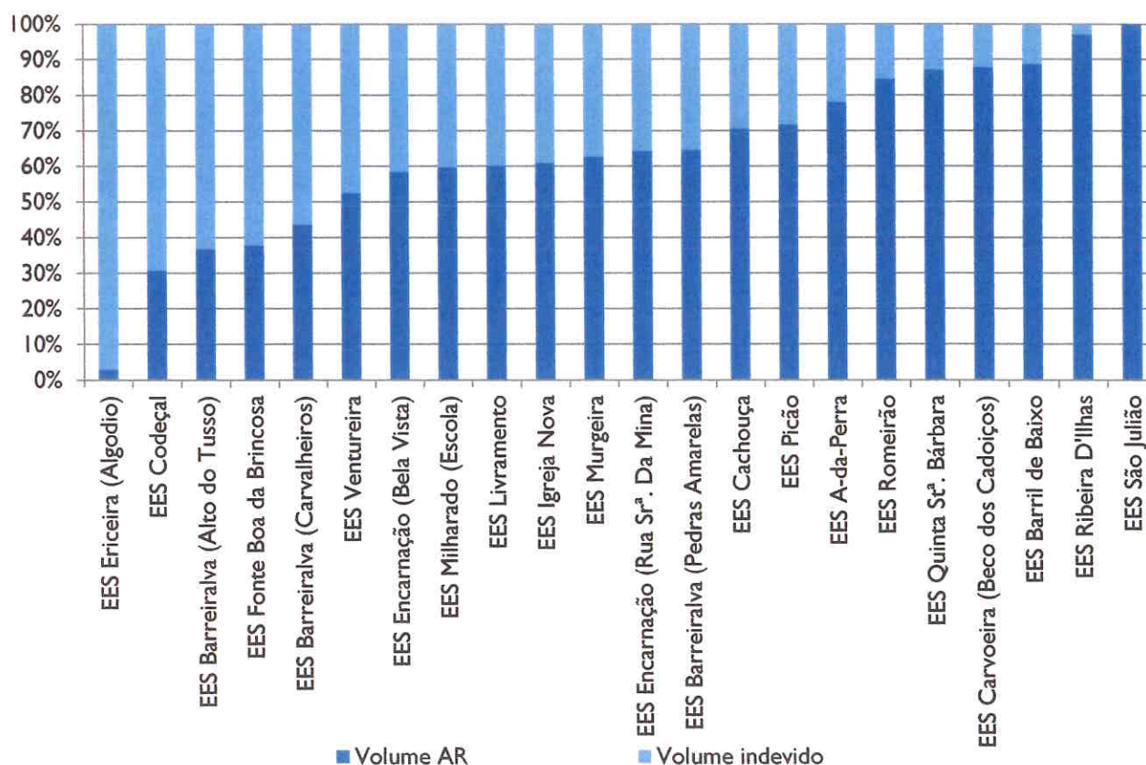
Gráfico 14 – Volumes das Estações Elevatórias
