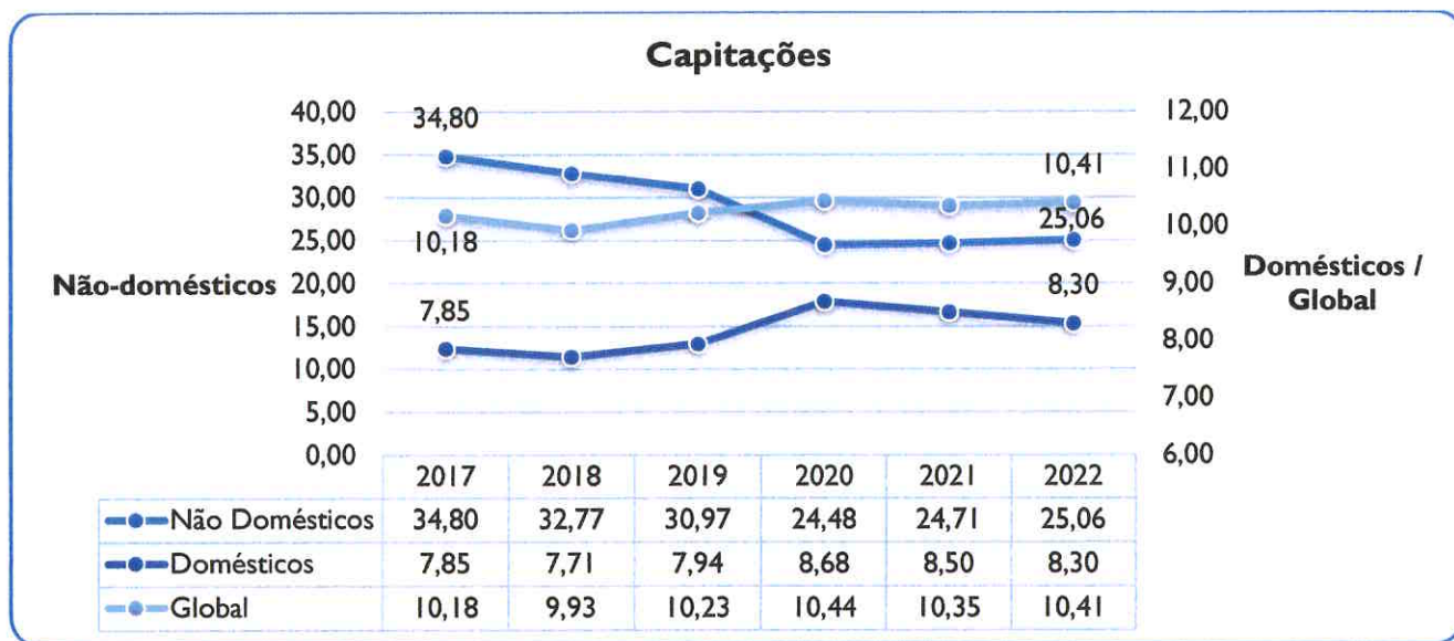
Gráfico 5 - Evolução das capitações de abastecimento de água
