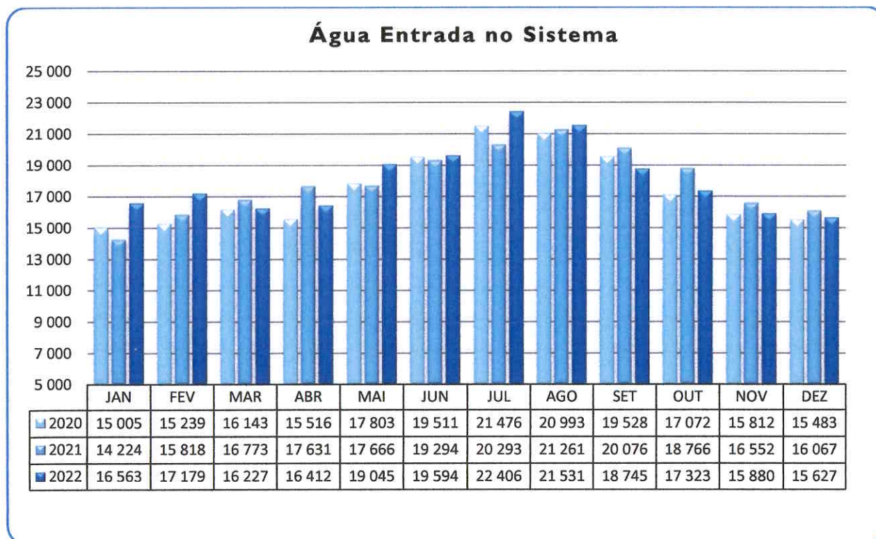
Gráfico 7 – Volume médio diário de água entrada no sistema
