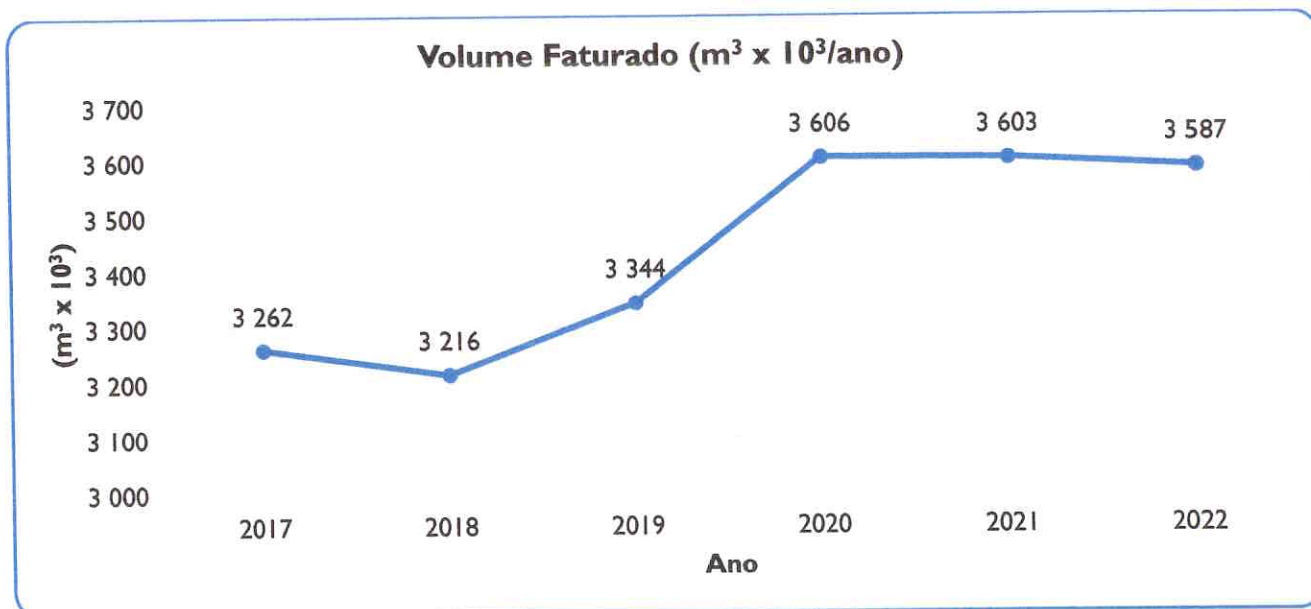
Gráfico 11 - Evolução do volume faturado de águas residuais
