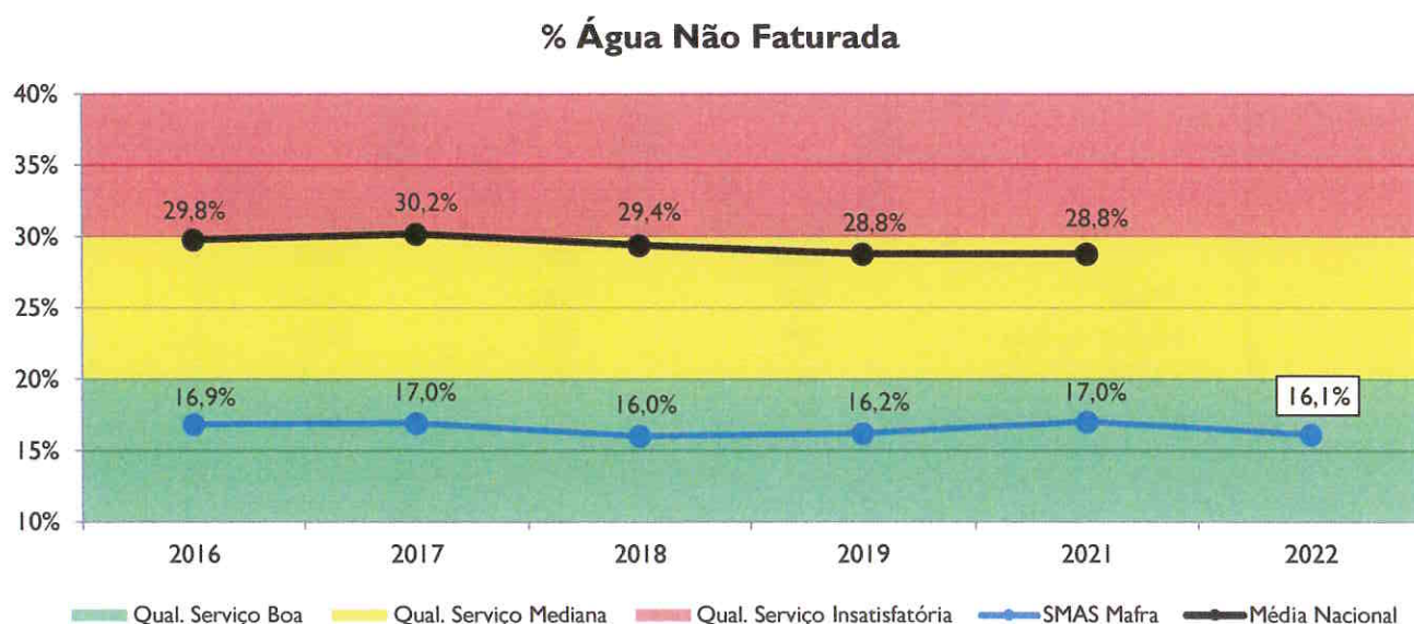
Gráfico 8 – Evolução da percentagem de água não faturada
