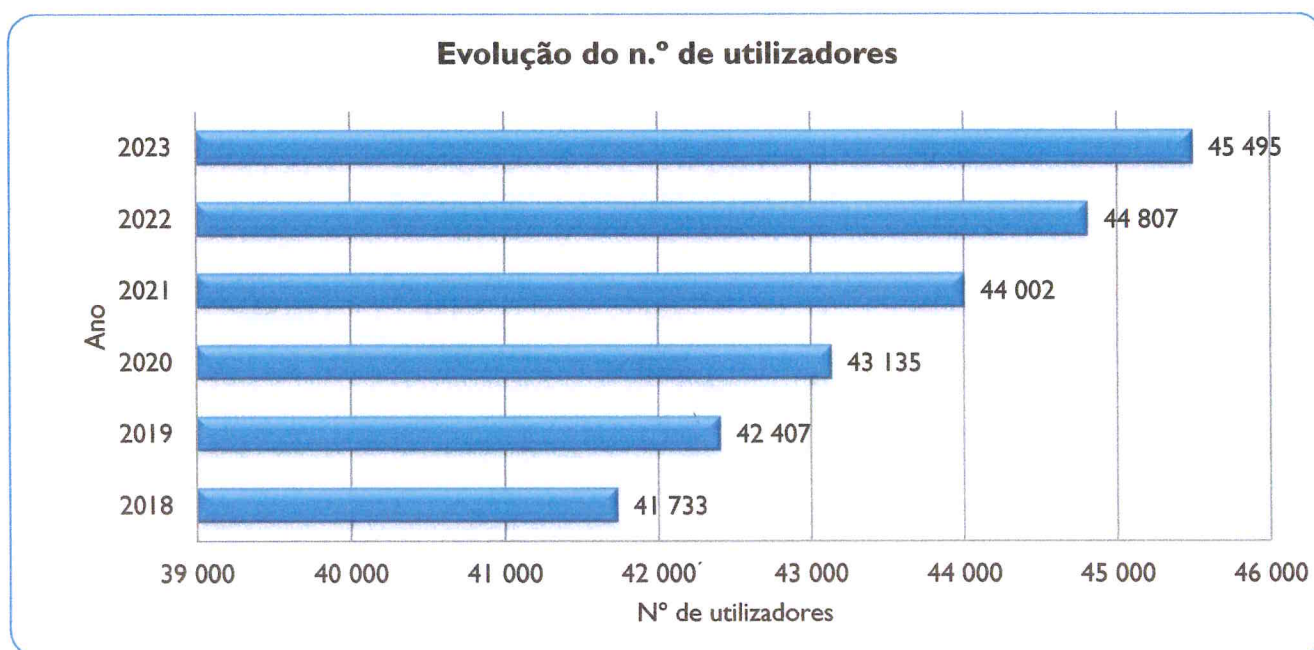
Gráfico 5 - Evolução do número de utilizadores do serviço de abastecimento de água
