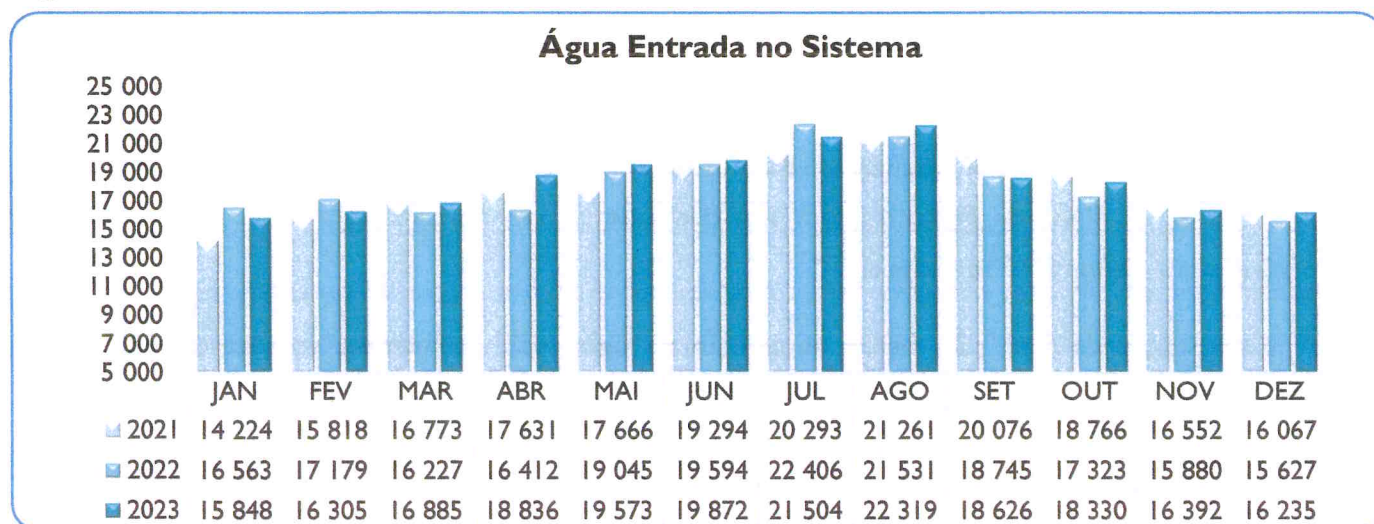
Gráfico 9 – Volume médio diário de água entrada no sistema
