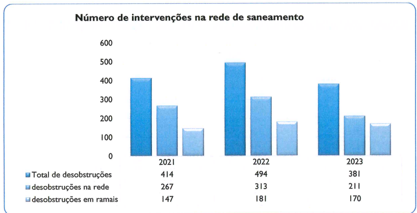
Gráfico 14 – Número total desobstruções e intervenções na rede de saneamento
