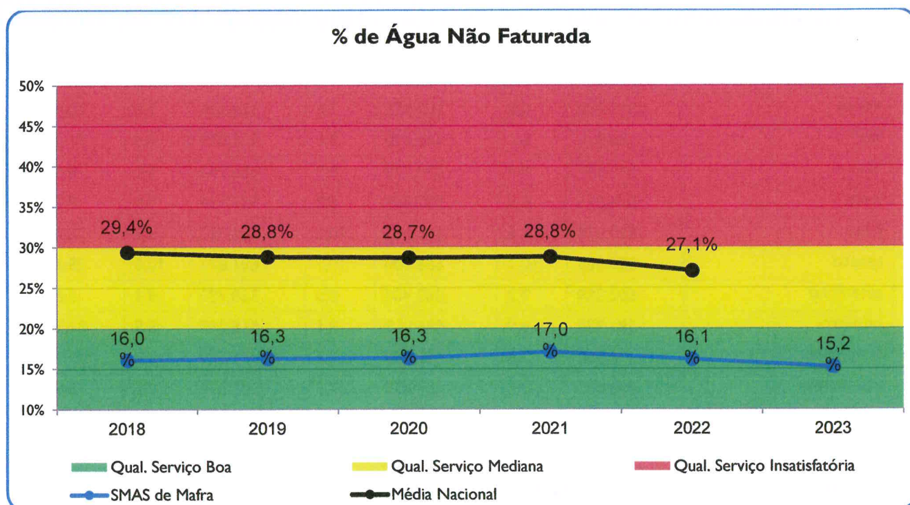
Gráfico 10 – Evolução da percentagem de água não faturada
