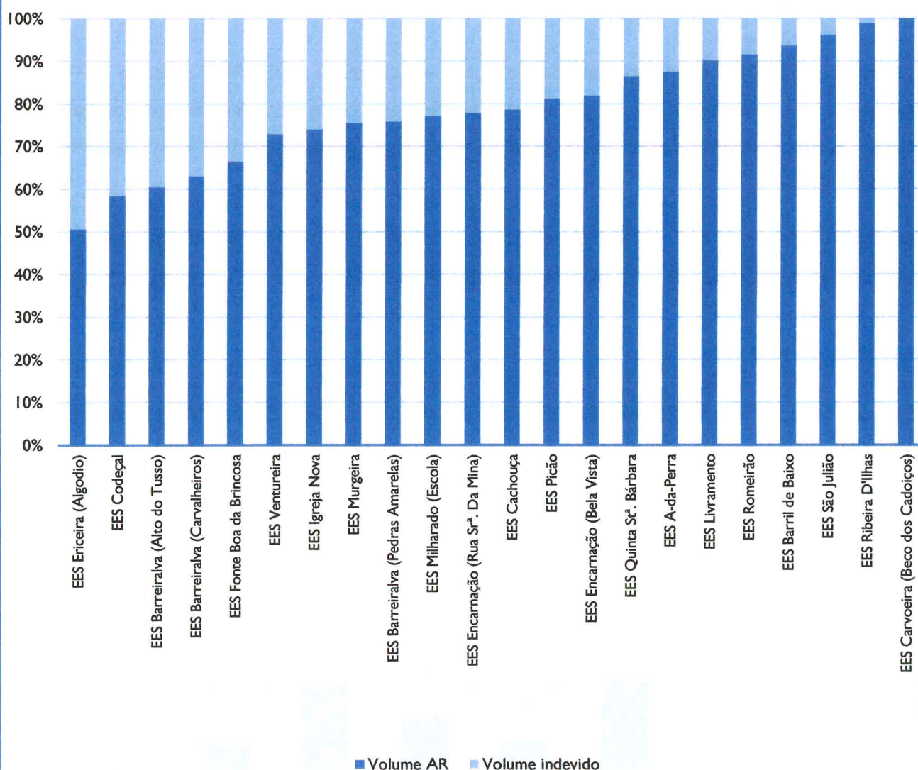
Gráfico 16 – Volumes das Estações Elevatórias
